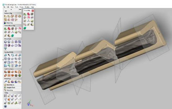
Figur 8. Freeform med guidning för hur fibulabenet sågas.
